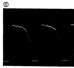
Q01-C 240Vp-p POWER OFF
