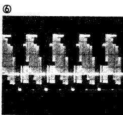
IC301-28 2.0Vp-p PB/REC
