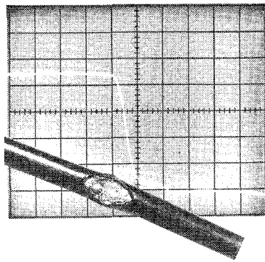
FIG. 2—A TEKTRONIX 1502 displays a short circuit.
