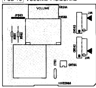
PCB-10 VOLUME P.C.BOARD
