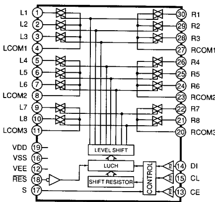
IC102 IC151 : LC7822 FUNCTION SELECTOR
