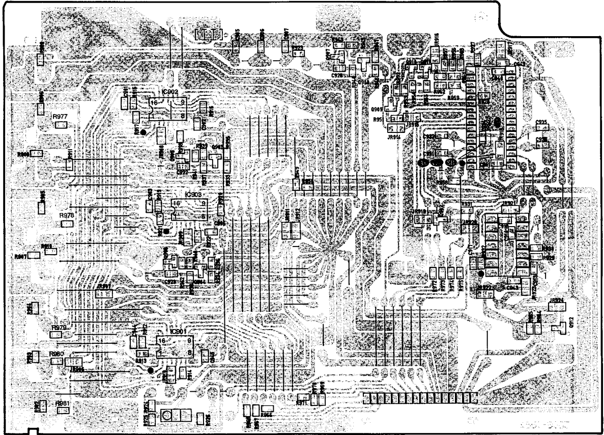
(Pattern Side)
